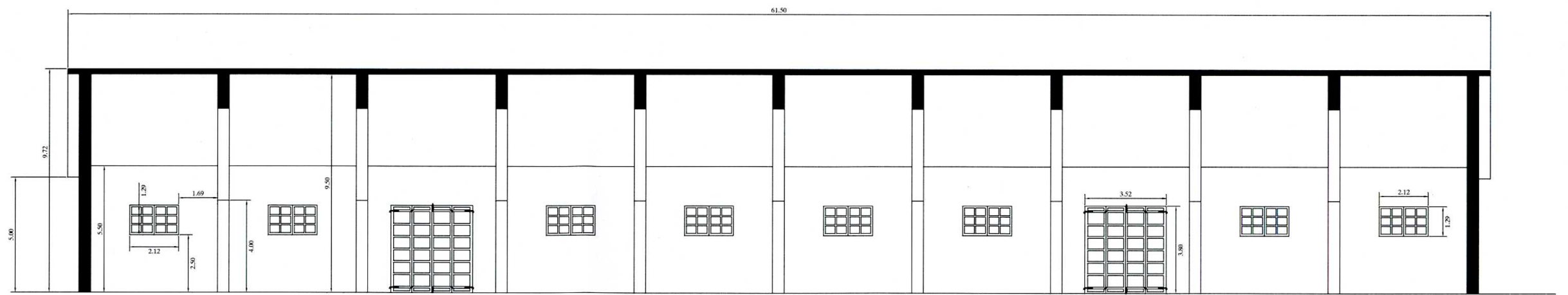
sezione longitudinale ovest
