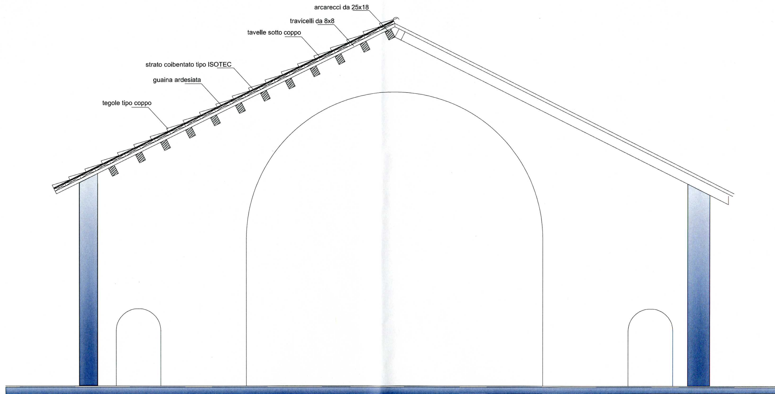
sezione copertura con particolare costruttivo
